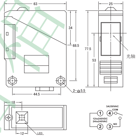
图192 HDT1000-36K-□ HDM100-36K-□ HDR400-36K-□
