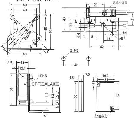
图187 HD-E3JK-5□ HD-E3JK-DS30□ HD-E3JK-R2□
