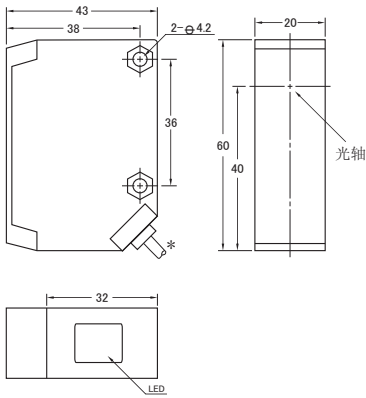
图189 HDT500-20K-□ HDM30-20K-□
