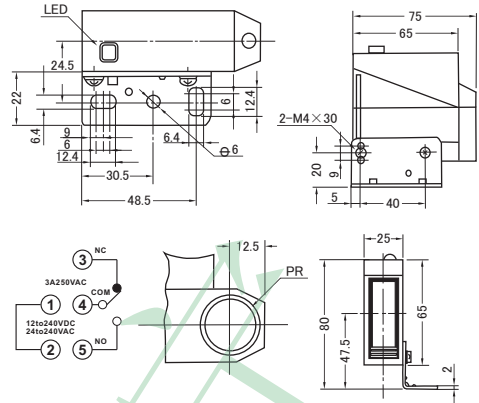
图190 HD-VT-5000□ HD-VD-80□ HD-VR-2000□
